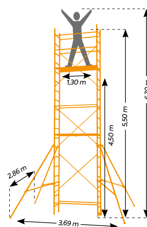
Speed'Up XL hauteur du plancher 4,5 m
